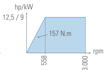
Broche ASA A2-6" – 3.000 rpm
