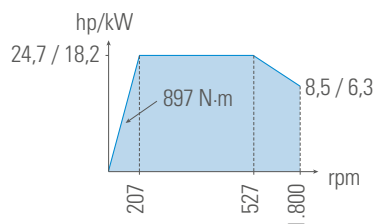
Broche ASA A2-8" – 1.800 rpm
