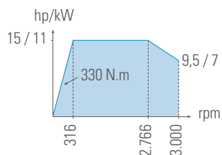
Broche ASA A2-6" – 3.000 rpm
